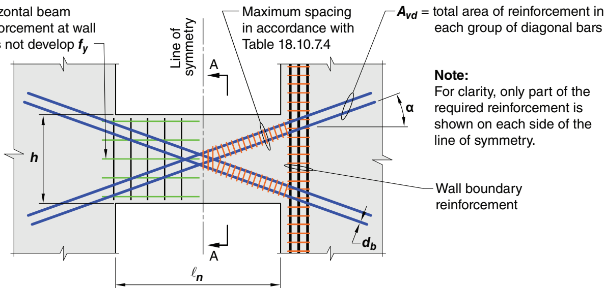
Elevation
