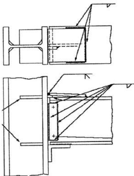
شکل ۱-۲۸- اتصال صلب تیر به ستون
