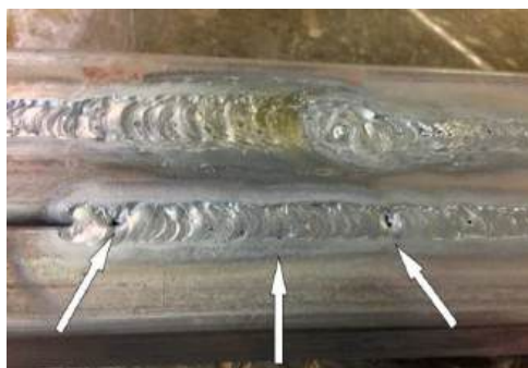
شکل ۱-۲۲- تخلخل جوش
