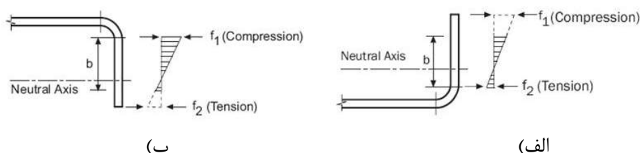
شکل ۲-۱۲ جزء سخت نشده، تحت فشار تحت تنش غیریکنواخت، یک لبه تحت فشار و لبه دیگر تحت کشش
