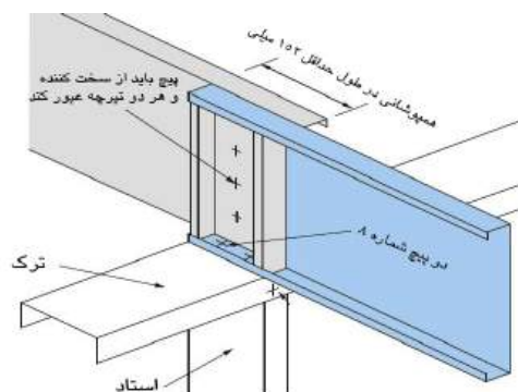
شکل ۷-۳۱ نمونه جزئیات اجرای وصله تیرچه بر روی تکیه‌گاه میانی
