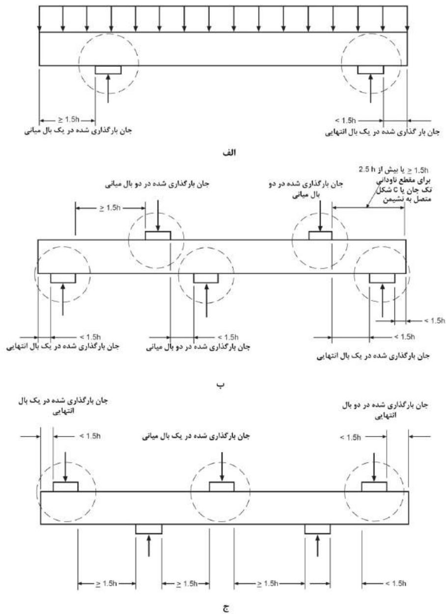
شکل ۳-۱ تعریف شرایط جان بارگذاری شده در دو بال و یک بال در حالت انتها و میان
