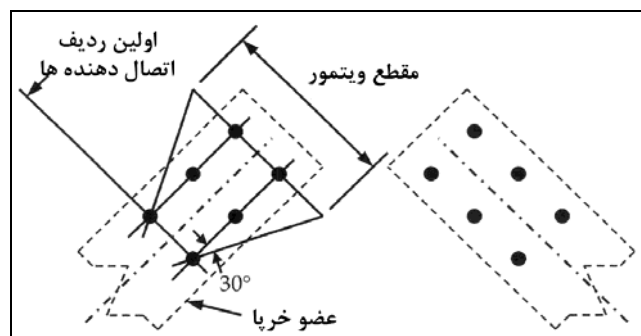
شکل ۴-۴ عرض ورق ویتور
