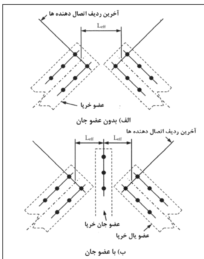
شکل ۴-۴ عرض ورق ویتور
