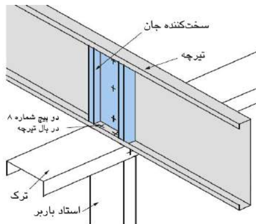
شکل ۷-۲۹ اجرای سخت کننده در تیرچه روی دیوار باربر میانی
