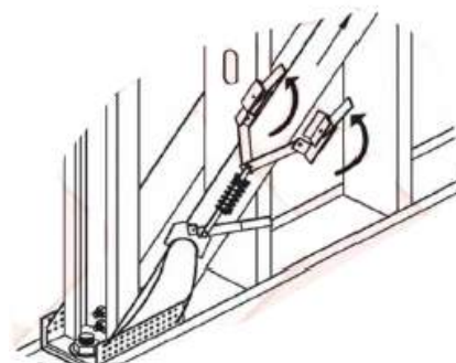
شکل ۲۶-۷ ابزار مورد استفاده برای ایجاد پیش کشیدگی اولیه در مهاربند تسمه‌ای قطری
