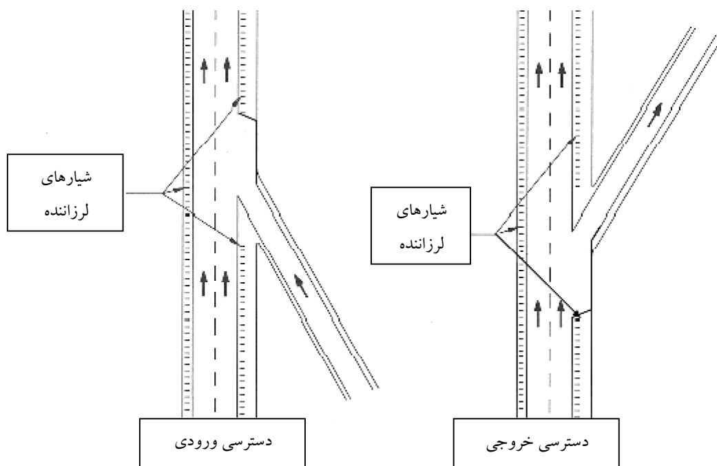
شکل شماره ۱: نحوه اجرای شیارهای لرزاننده کناری در راهها، موضوع بند ۱-۵
