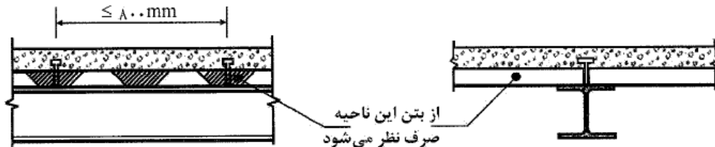
شکل ۱۰-۲-۸-۵ ورق‌های فولادی شکل داده شده که کنگره‌های آنها عمود بر محور تیر می‌باشد
