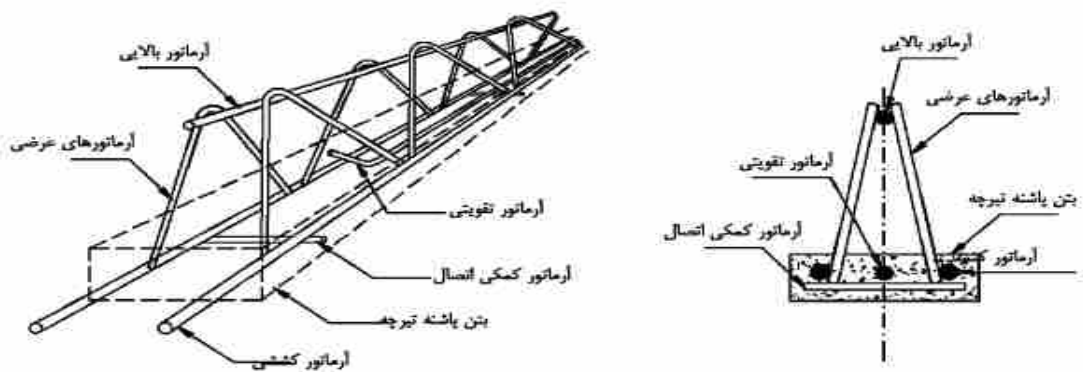
شکل ۸-۱- اجزای تیرچه پیش ساخته خربایی
