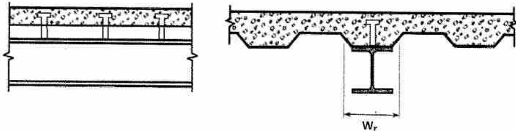
شکل ۶-۸-۲-۱۰ ورق‌های فولادی شکل داده شده که کنگره‌های آنها موازی با محور تیر می‌باشد
