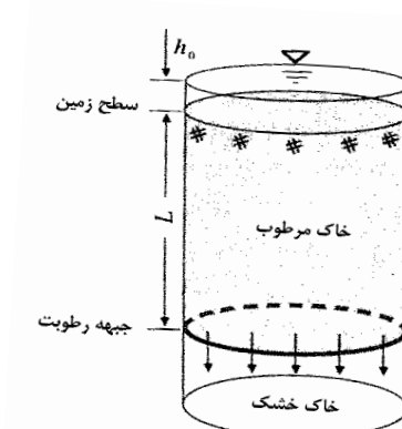
شکل (۷-۶) حرکت جبهه رطوبت
