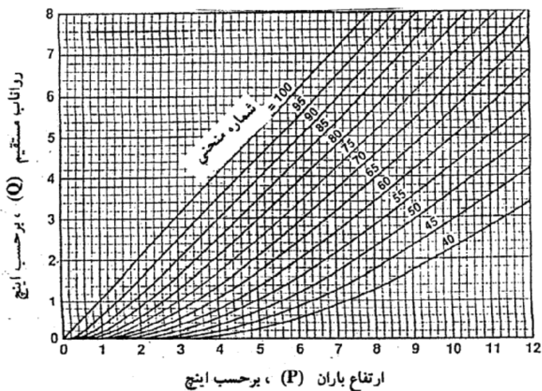
شکل (۳-۹) رابطه بین بارش تجمعی و روان آب تجمعی برای مقادیر مختلف CN
