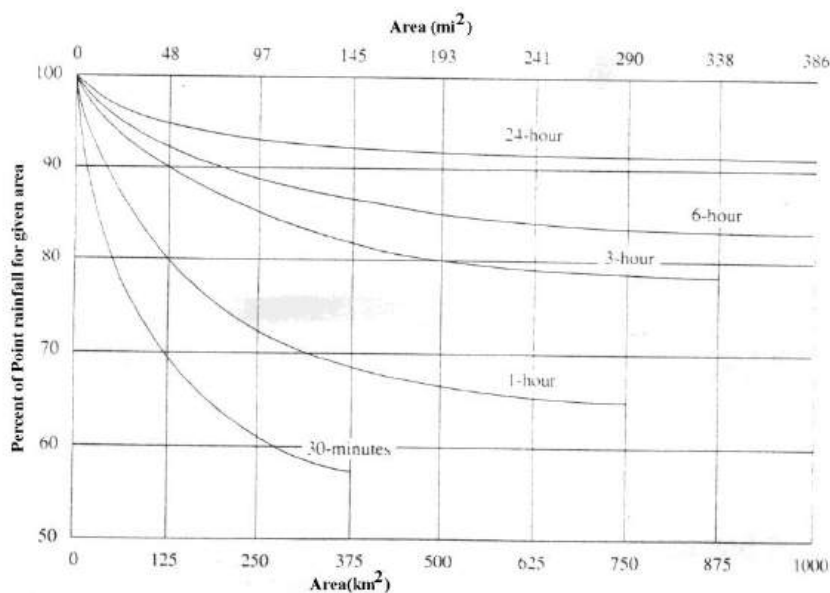
شکل (۴-۱۸) یک منحنی ضریب کاهش سطح
