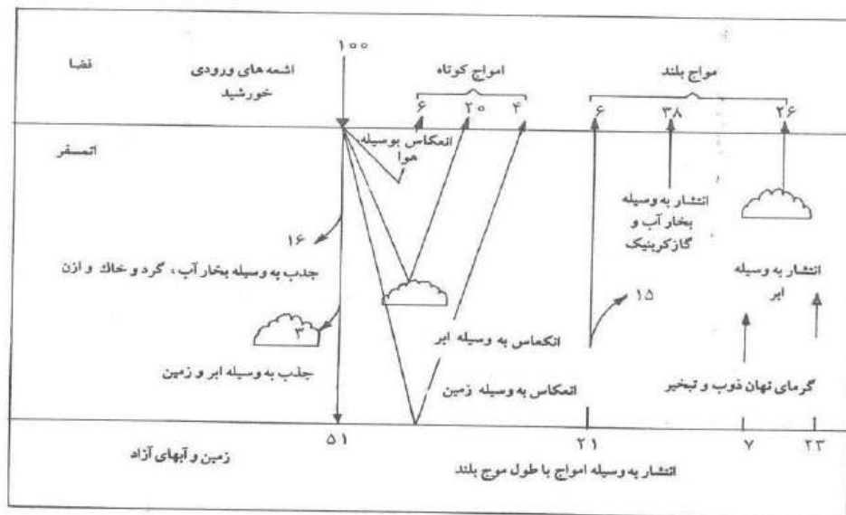
شکل (۲-۳) مؤلفه های بیلان حرارتی زمین و اتمسفر
