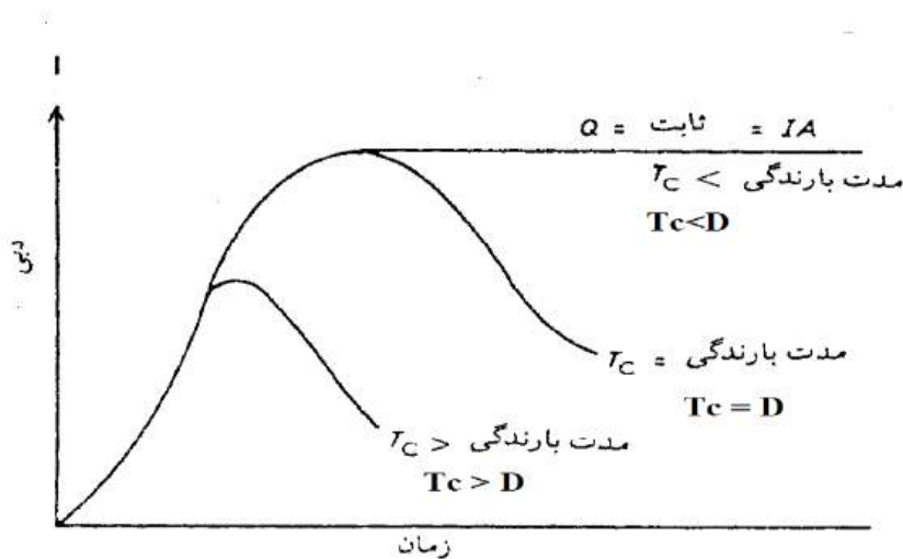
شکل ۷-۱۰- هیدروگراف حوضه با فرض یکنواخت بودن بارش
