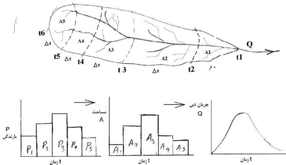
شکل 10-1- روش مدت - مساحت
