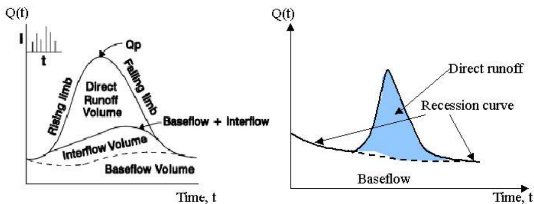
شکل (۱۱-۲) کسر جریان پایه از هیدروگراف مشاهداتی و تعیین حجم رواناب مستقیم
