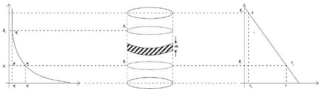
شکل (۹-۲) تغییرات فشار و درجه حرارت نسبت به هوا
