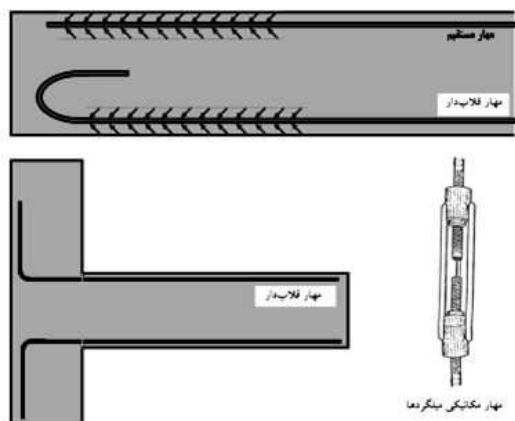
روشهای مختلف مهار میلگرد در بتن
