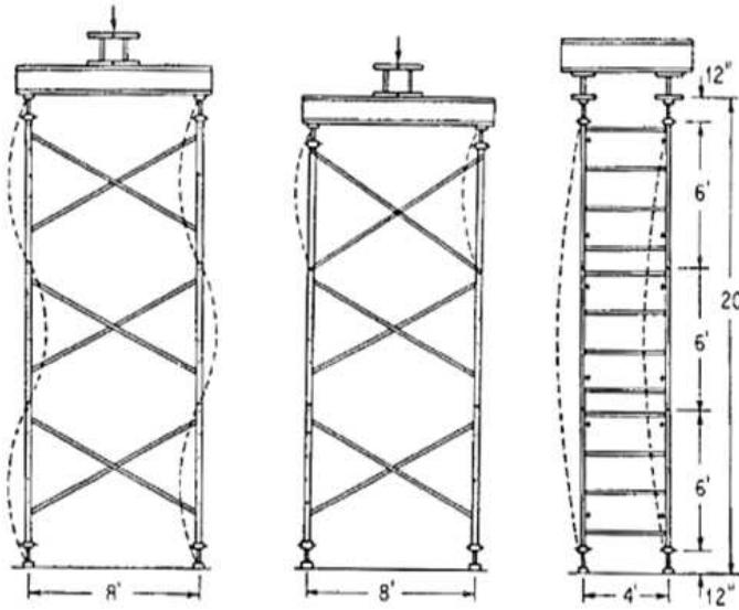
مودهای مختلف کمانشی داربست ها.
