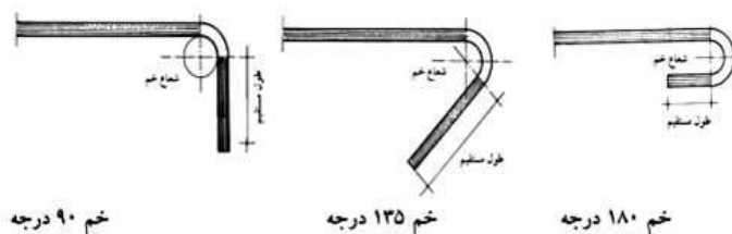
انواع شکل خم میلگرد
