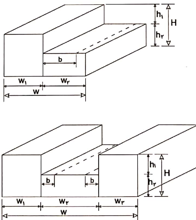
شکل ۱۰-۱۰-۶ نسبت ابعادی ساختمان‌های با بام پله‌ای تخت
