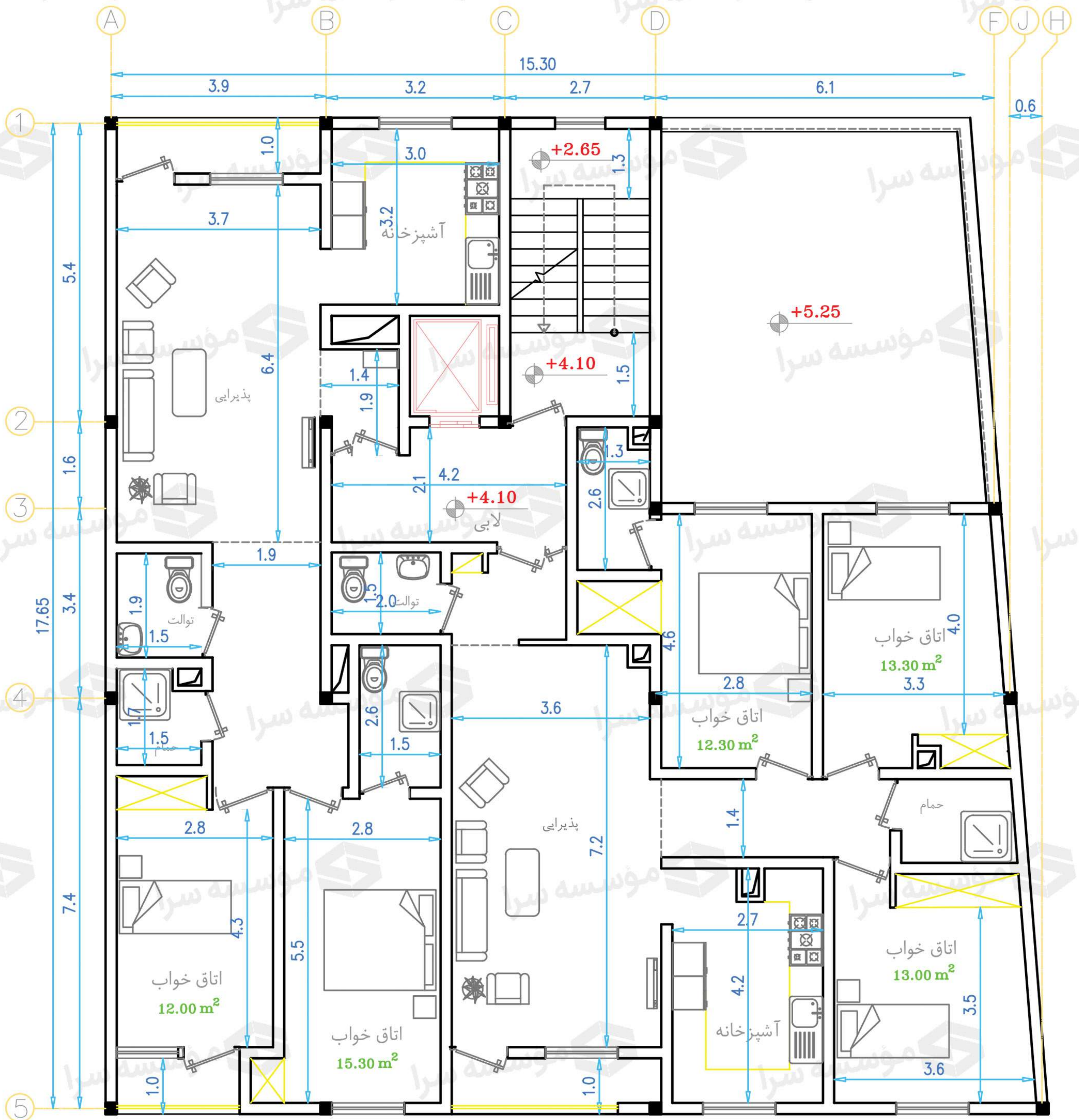
پلان طبقه یکم/ طراحی: دکتر اکرم خدای مدرس دوره های طراحی نظام مهندسی ساختمان
