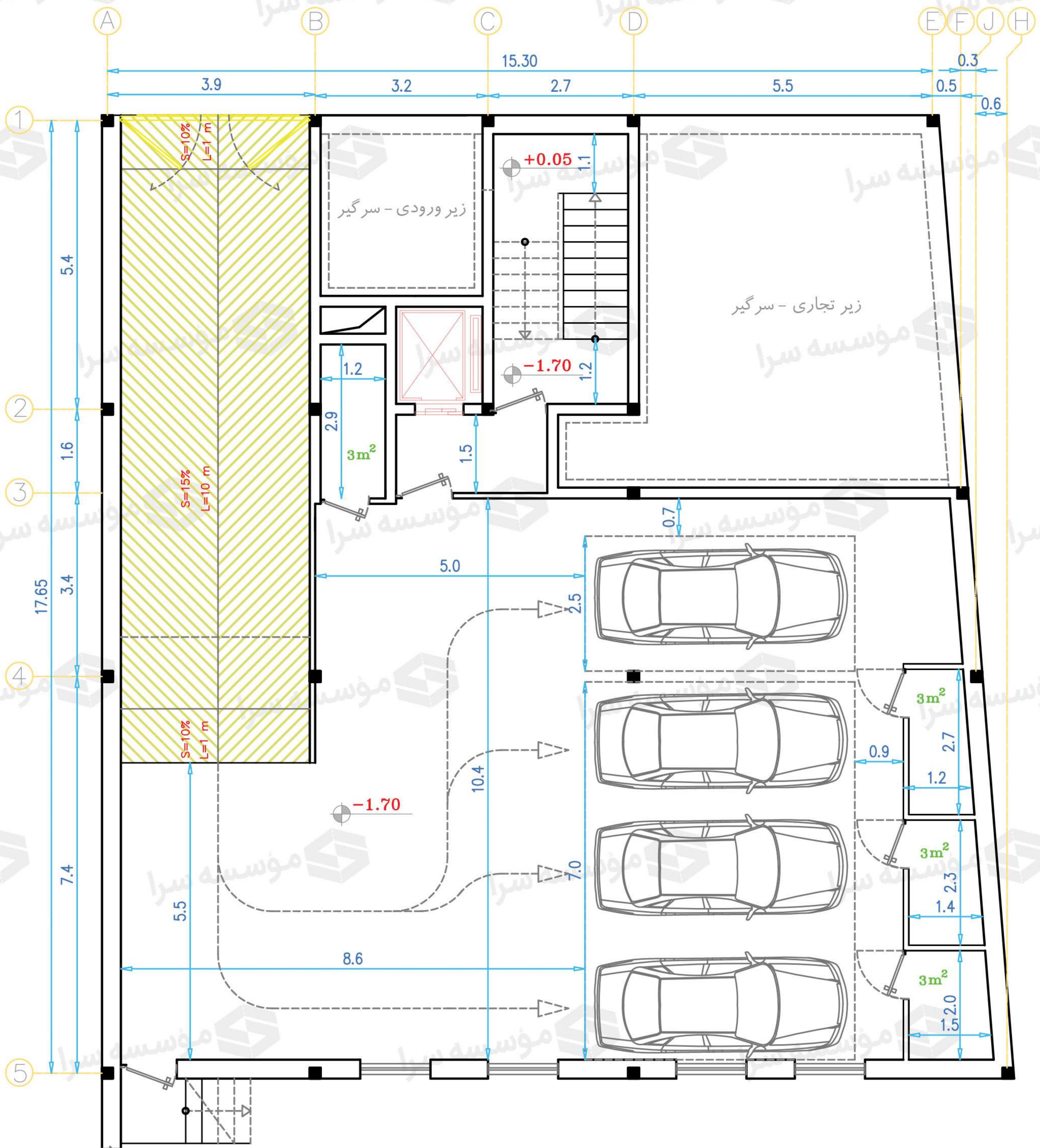
پلان طبقه زیرزمین / طراحی: دکتر اکرم خدای مدرس دوره های طراحی نظام مهندسی ساختمان
