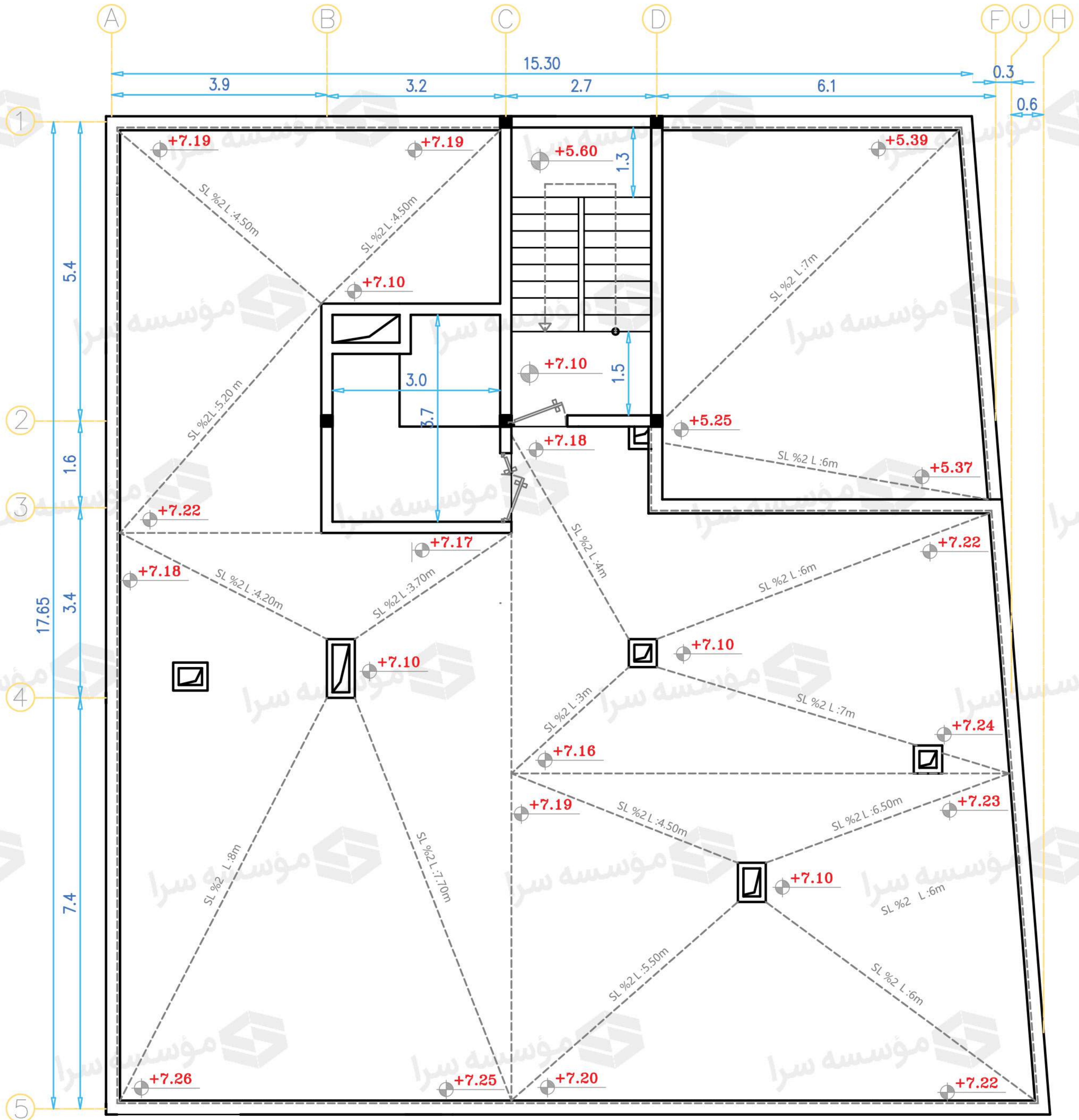
پلان بام / طراحی: دکتر اکرم خدای مدرس دوره های طراحی نظام مهندسی ساختمان
