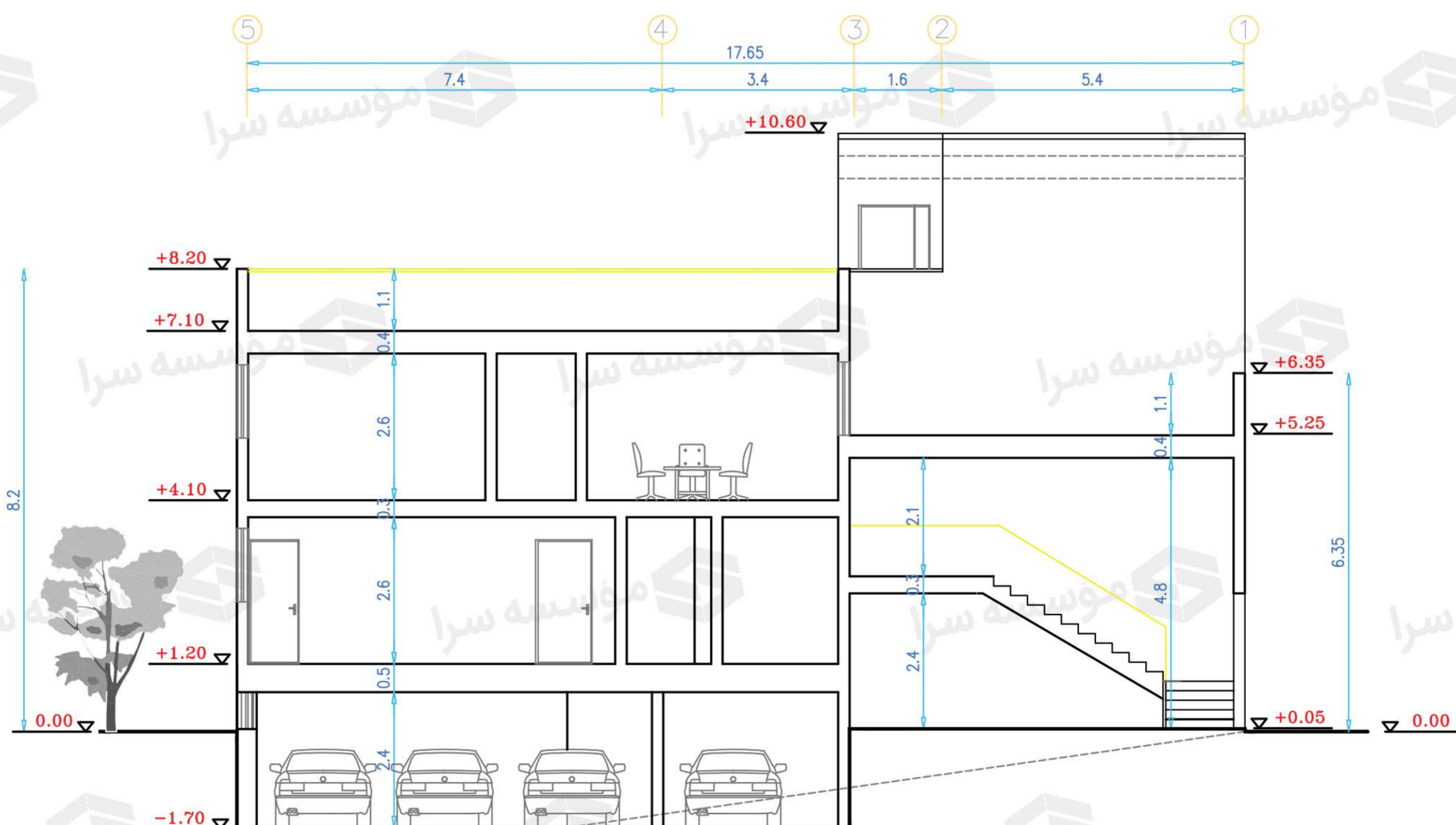
مقطع بنا / طراحی: دکتر اکرم خدایي مدرس دوره های طراحی نظام مهندسی ساختمان
