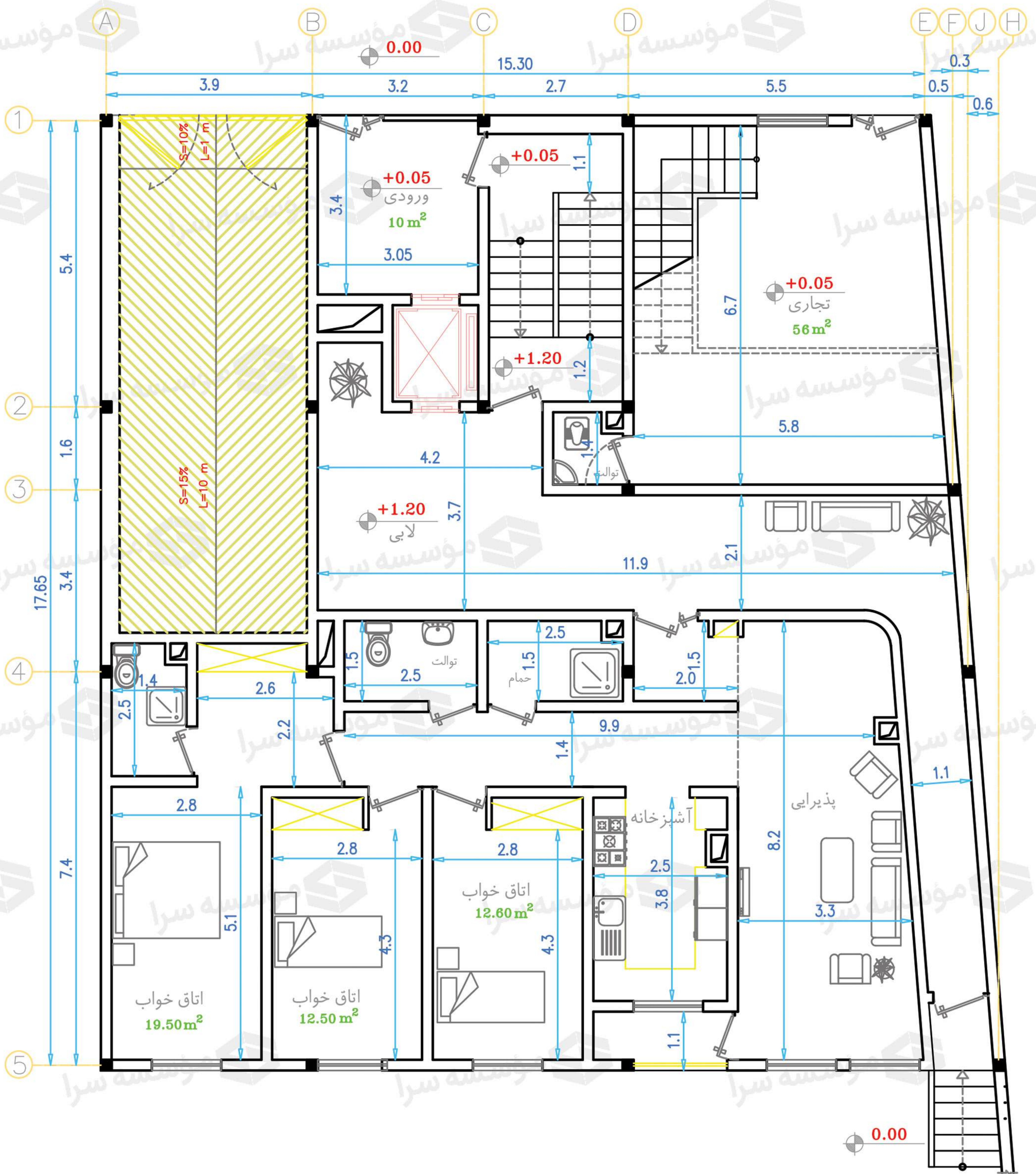
پلان طبقه همکف / طراحی: دکتر اکرم خدای مدرس دوره های طراحی نظام مهندسی ساختمان
