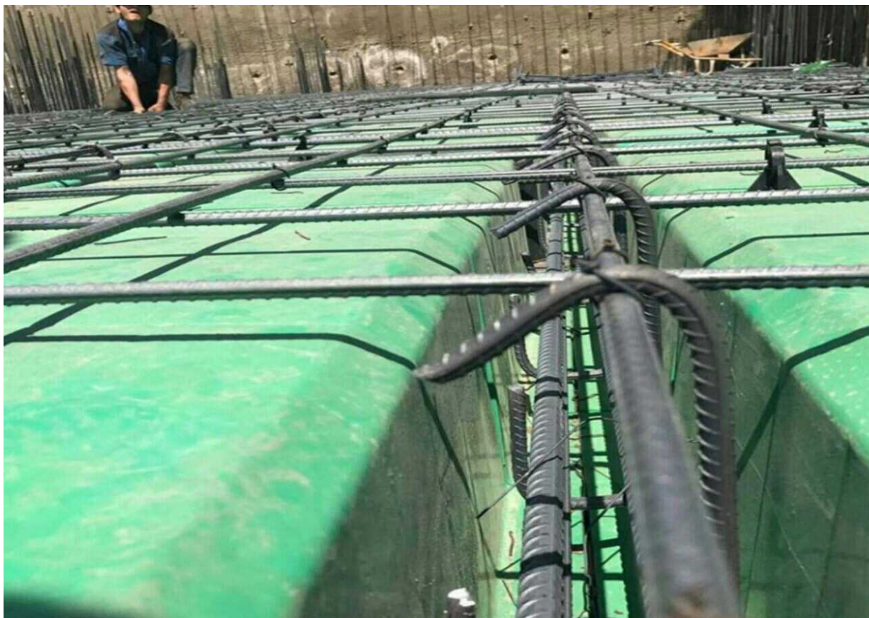
اجرای تیرچه درجا با حذف خرپا
