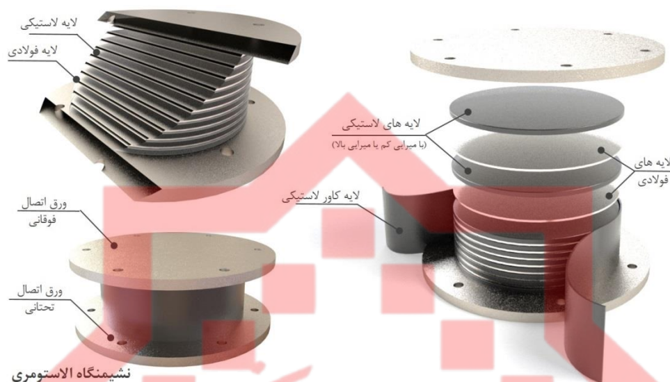
شکل (۳-۱). جزئیات نشیمنگاه‌های لاستیکی با میرایی کم و میرایی بالا
