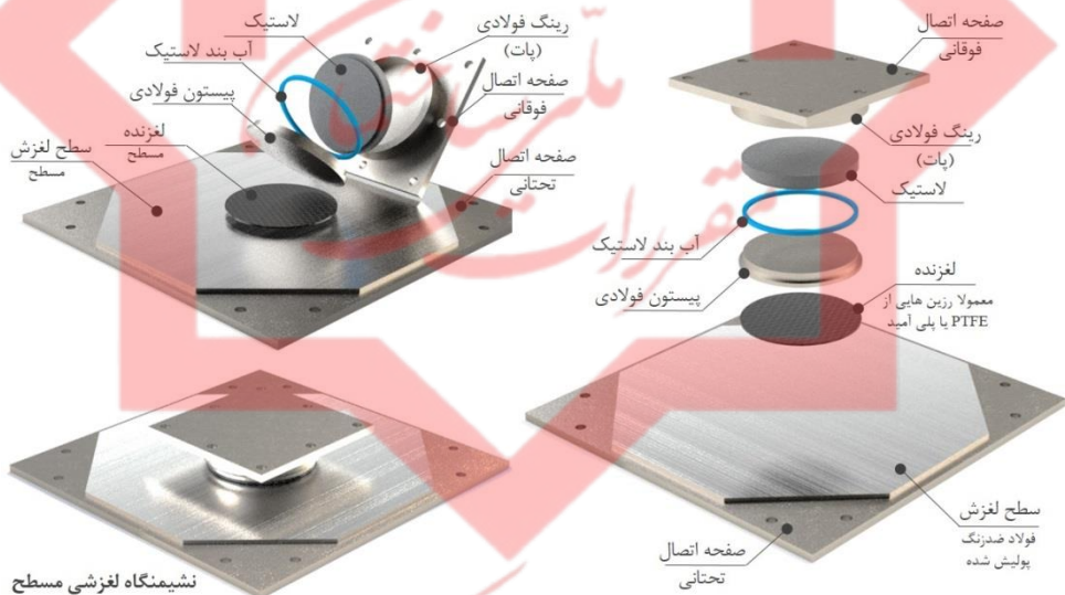
شکل (۱۱-۳). جزئیات نمونه‌ای از نشیمنگاه‌های لغزشی مسطح
