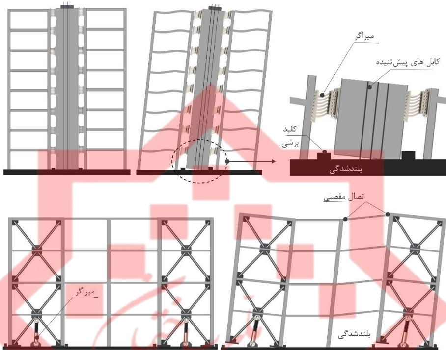
شکل (۲-۵۵). چیدمان گهواره‌ای میراگرها در ساختمان
