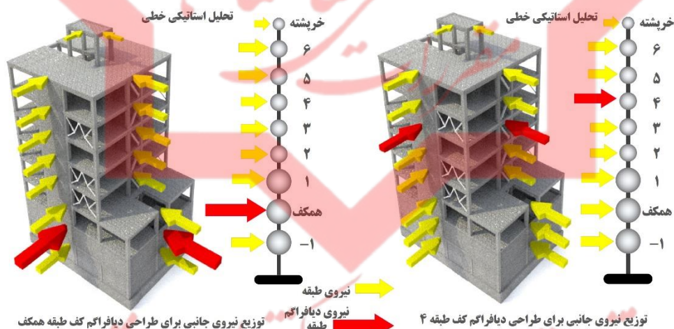
شکل (۷-۱۱). نمونه‌ای از بارگذاری سازه به منظور طراحی دیافراگم کف
