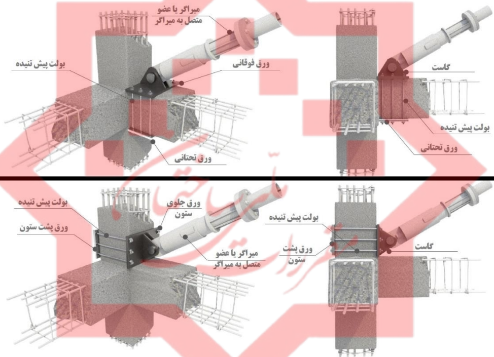
شکل (۷-۴). نمونه‌ای از اتصالات مقید نشده برای میراگرهای با عملکرد محوری در سازه‌های بتنی
