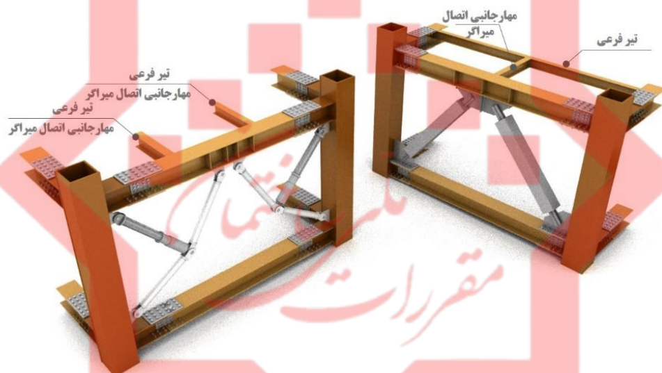
شکل (۷-۷). مهار جانبی در محل اتصال میراگر به میانه تیر
