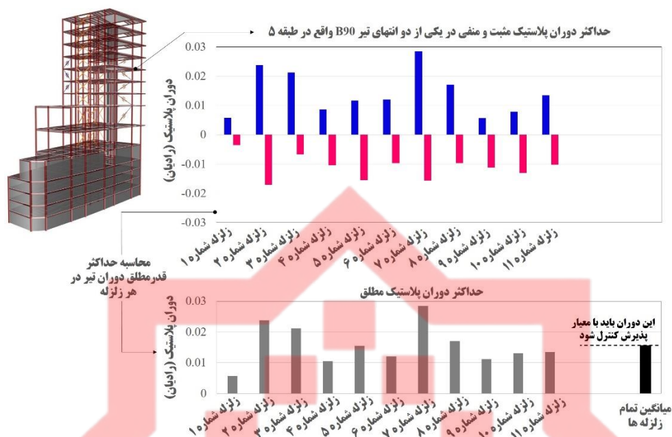
شکل (۵-۲۴). نمونه‌ای از نحوه محاسبه میانگین حداکثر دوران پلاستیک تیر فولادی حاصل از تمام زلزله‌ها
