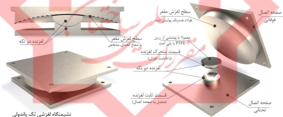
شکل (۳-۱۴). جزئیات نمونه‌ای از نشیمنگاه‌های لغزشی تک پاندولی
