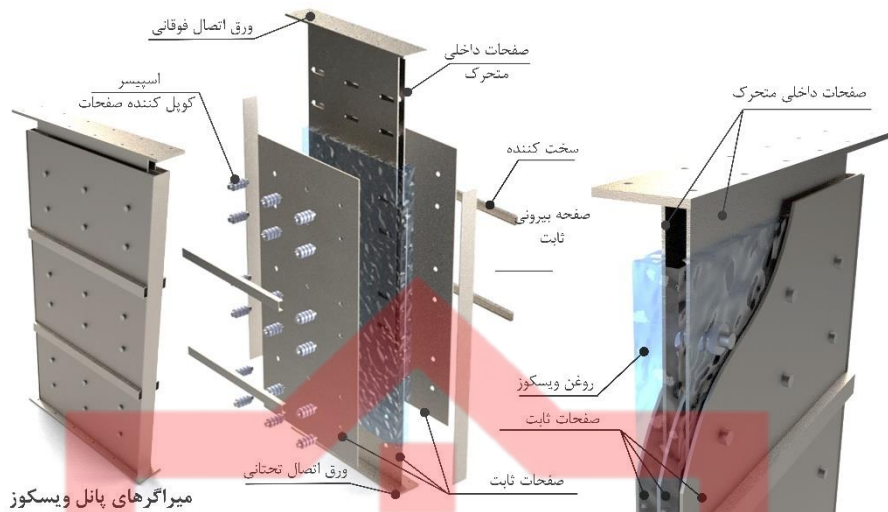
شکل (۲-۳۲). جزئیات نمونه‌ای از میراگرهای پانل ویسکوز
