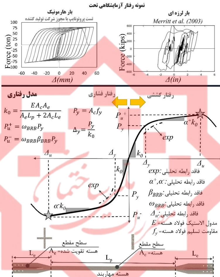
شکل (۲-۱۱). رفتار آزمایشگاهی مهاربندهای کماتش‌تاب و منحنی پوش رفتار آن‌ها
