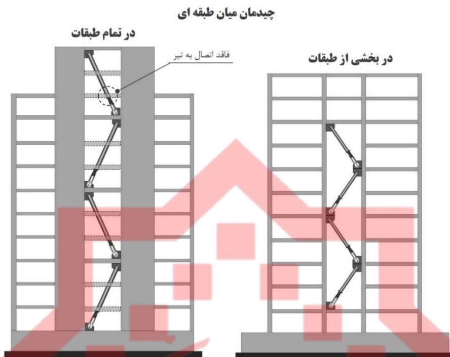
شکل (۲-۵۳). چیدمان میان طبقه ای میراگرها در ساختمان
