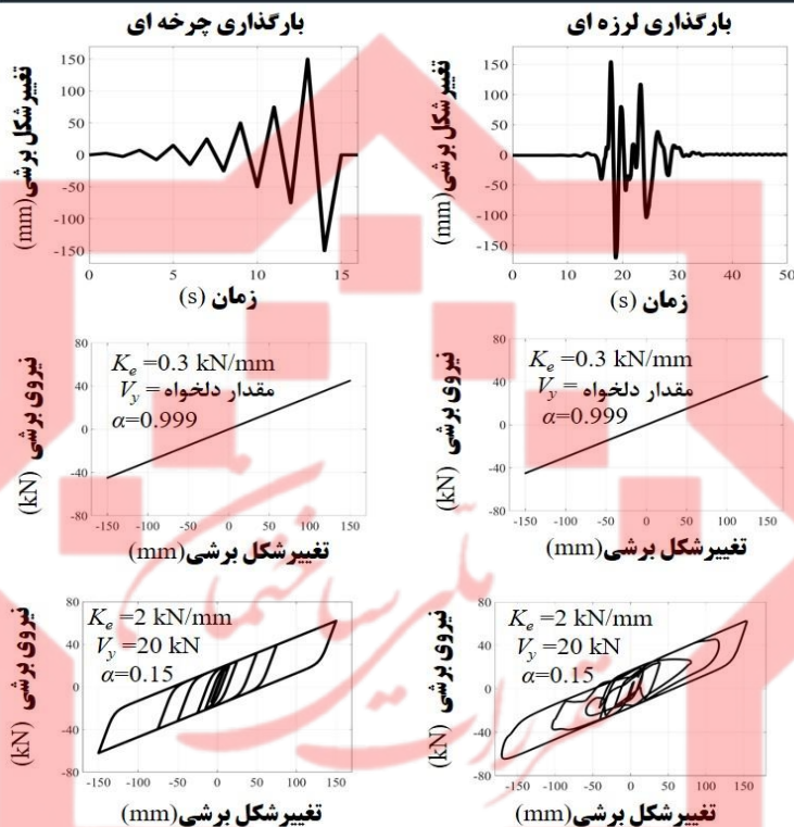
شکل (۳-۱۰). نمونه‌ای از نتایج شبیه سازی رفتار نشیمنگاه‌های لاستیکی با استفاده از رفتار برشی دوخطی (مقادیر استفاده شده برای کمیت‌های مدل صرفاً به منظور نمایش رفتار مدل عددی هستند).
