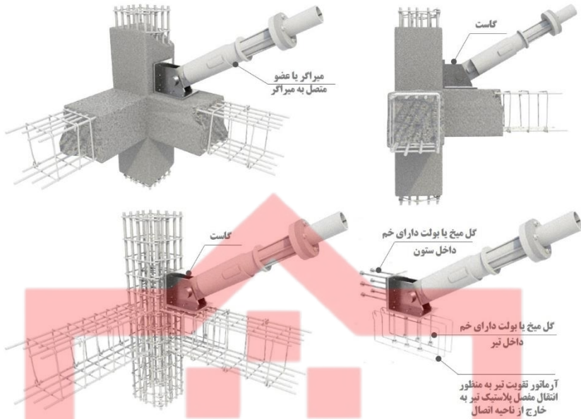
شکل (۷-۱). نمونه‌ای از اتصال میراگرهای با عملکرد محوری در سازه‌های بتنی جدید
