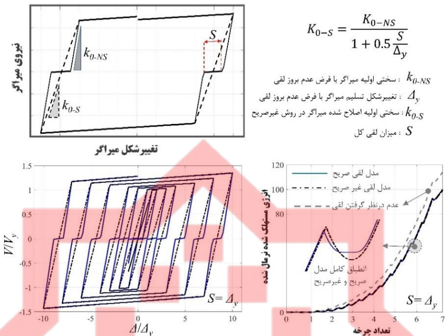
شکل (۲-۱۶). نحوه محاسبه سختی اولیه کاهش یافته میراگر تسلیمی به منظور در نظر گرفتن تاثیر لقی به صورت غیر صریح و مقایسه نتایج حاصل از مدل سازی صریح و غیر صریح لقی
