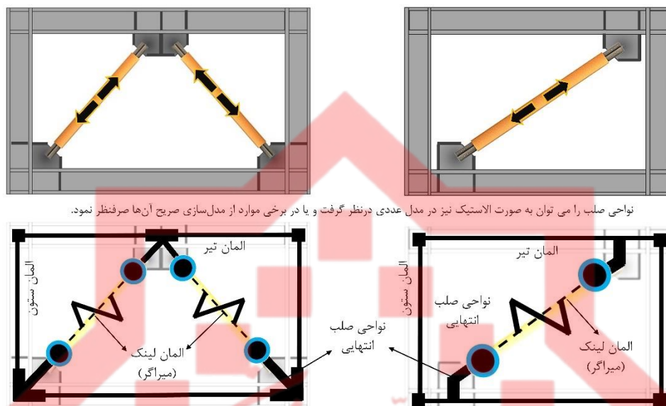
شکل (۲-۱۲). چیدمان‌های متداول برای استفاده از مهاربندهای کمناش تاب و نحوه مدل‌سازی آن‌ها
