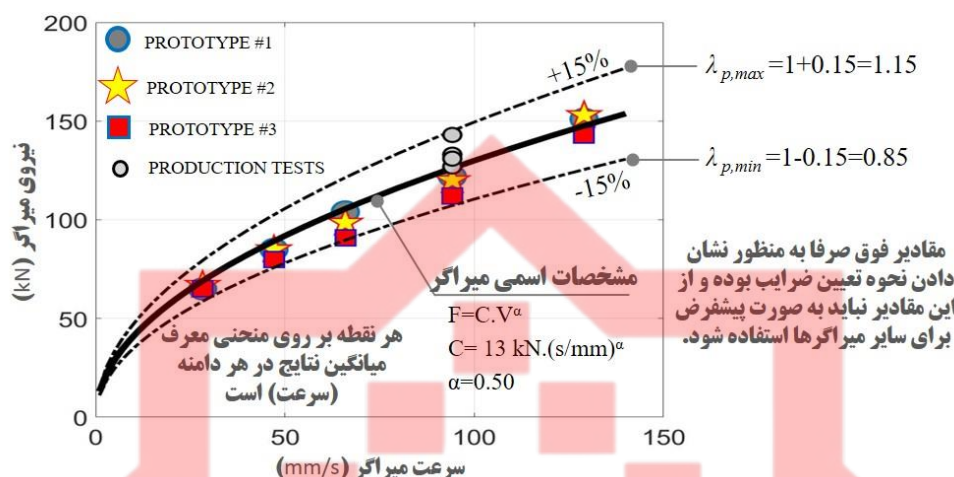
شکل (۴-۶). نمونه‌ای از محاسبه ضرایب \lambda_{p,min} و \lambda_{p,max} بر اساس نتایج حاصل از آزمایش‌های پروتوتایپ و کنترل محصول
