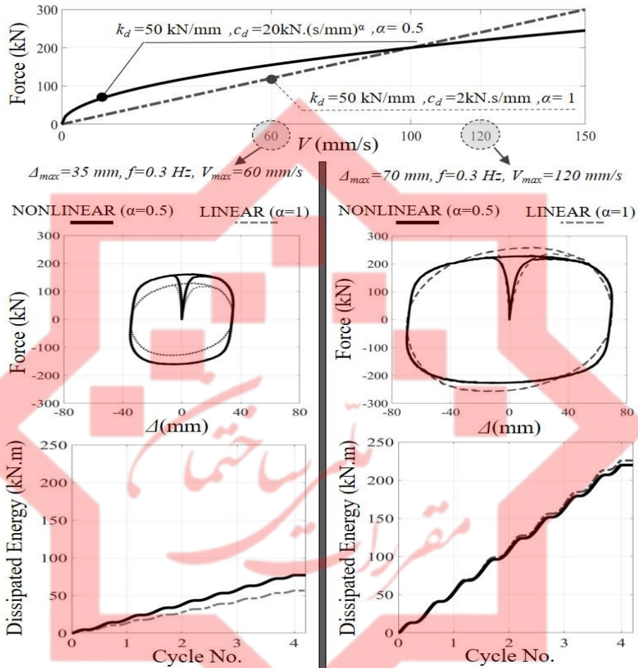
شکل (۲-۳۷). تاثیر توان سرعت میراگر در رفتار چرخه‌ای و میزان انرژی مستهلک شده در دو سرعت مختلف
