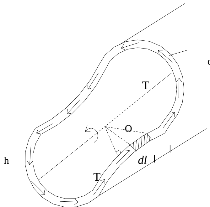
شکل ۱ - جریان برشی در قوطی جدار نازک
