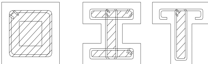
شکل ۳ - تعریف A_{oh} (سطح هاشور خورده)
