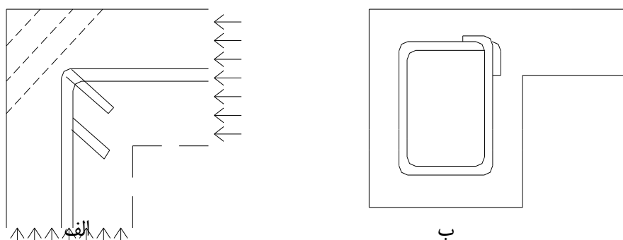
شکل ۸ - فروریختگی گوشه تیر ناشی از بار پیچشی
